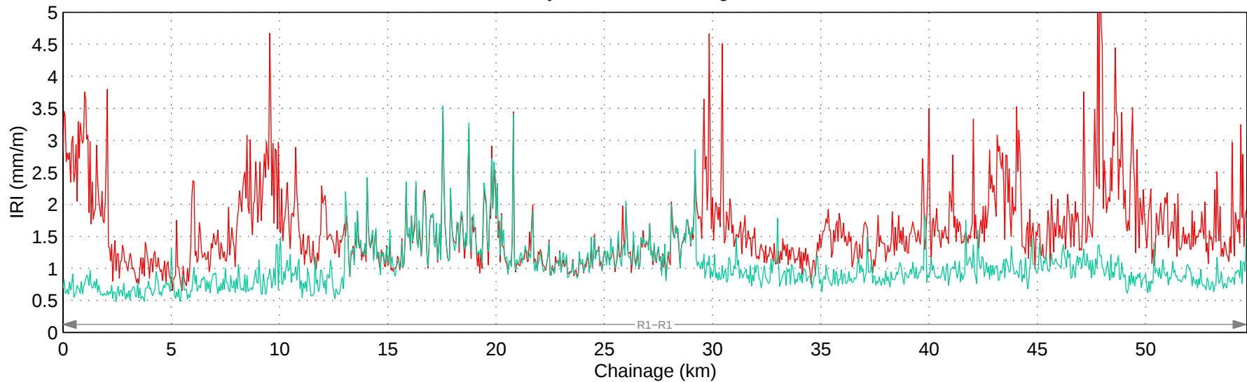
Hwy 1:16 Mean IRI – Right Lane
