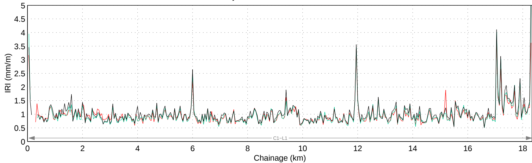
Hwy 596:02 Mean IRI – Left Lane
