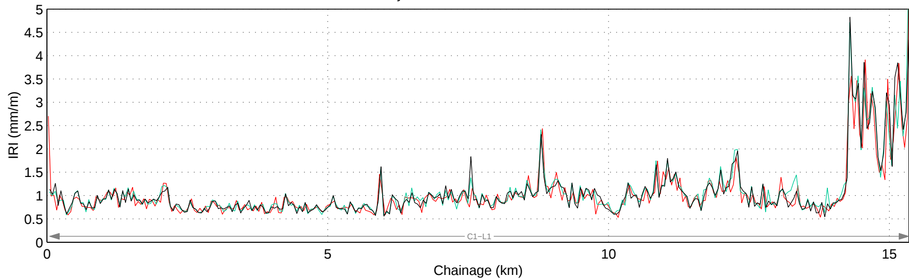
Hwy 546:02 Mean IRI – Left Lane
