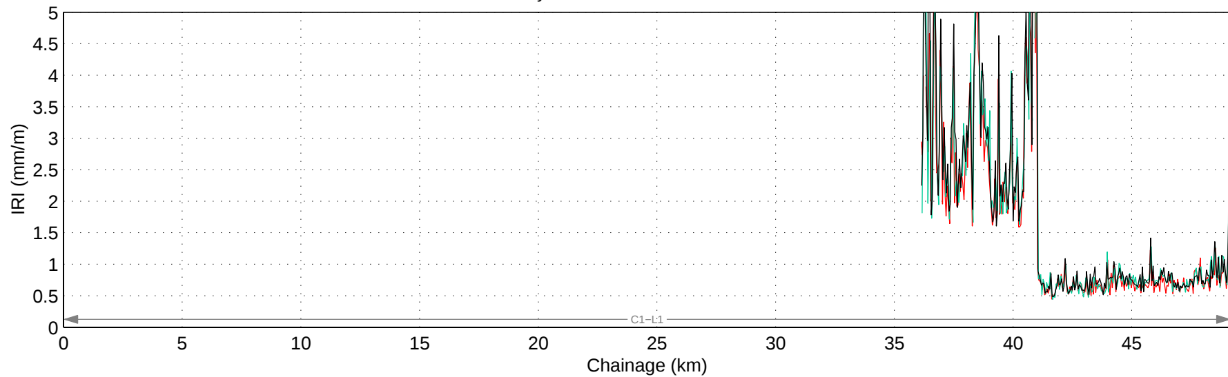
Hwy 579:02 Mean IRI – Left Lane
