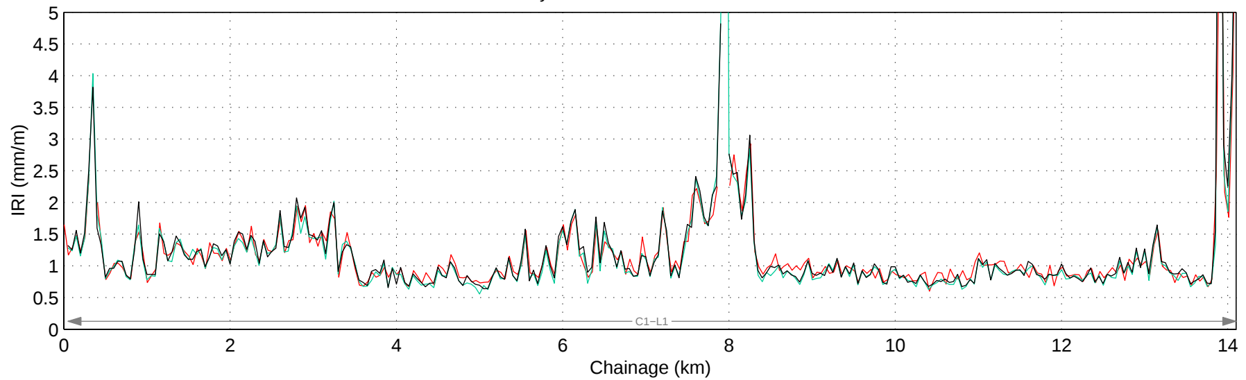
Hwy 527:02 Mean IRI – Left Lane
