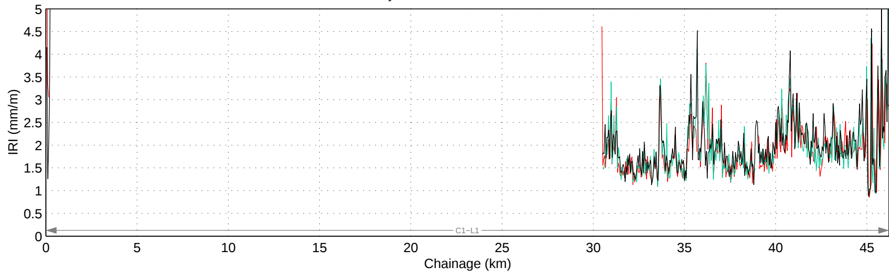
Hwy 520:02 Mean IRI – Left Lane
