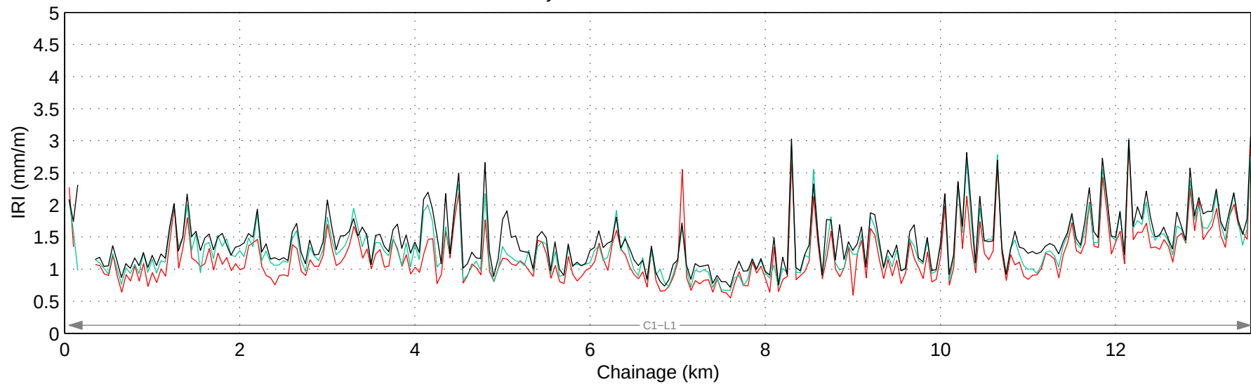
Hwy 719:02 Mean IRI – Left Lane
