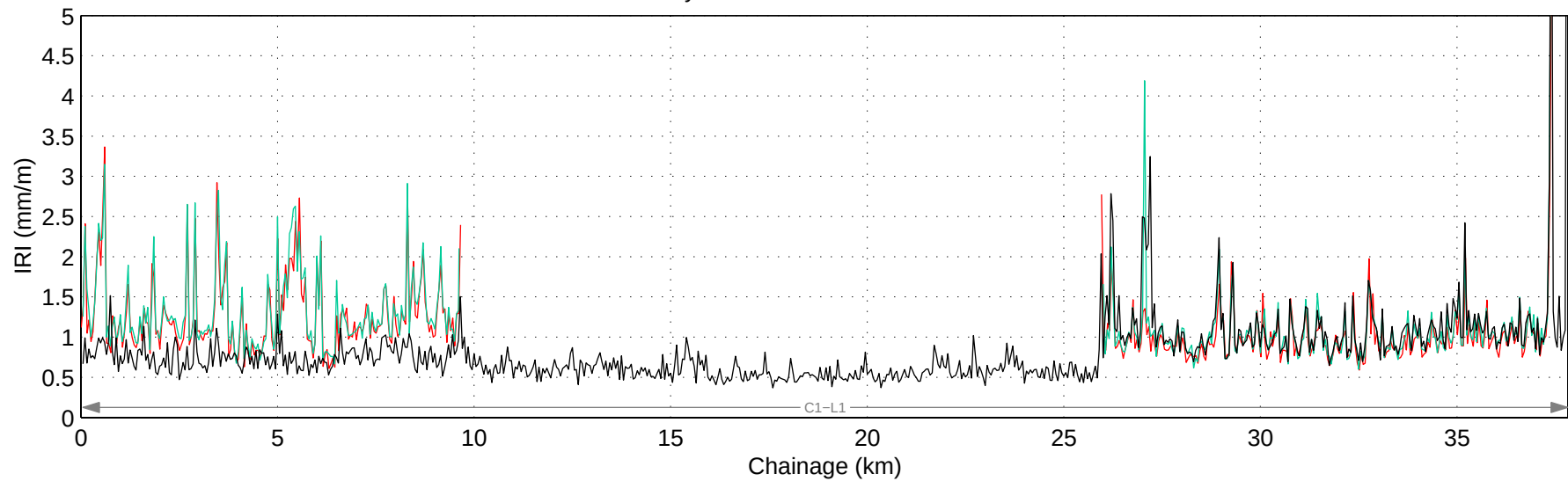
Hwy 753:04 Mean IRI – Left Lane
