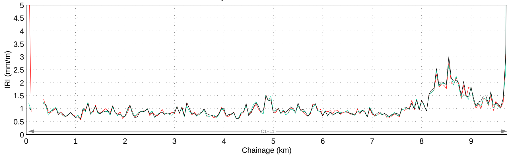
Hwy 770:02 Mean IRI – Left Lane
