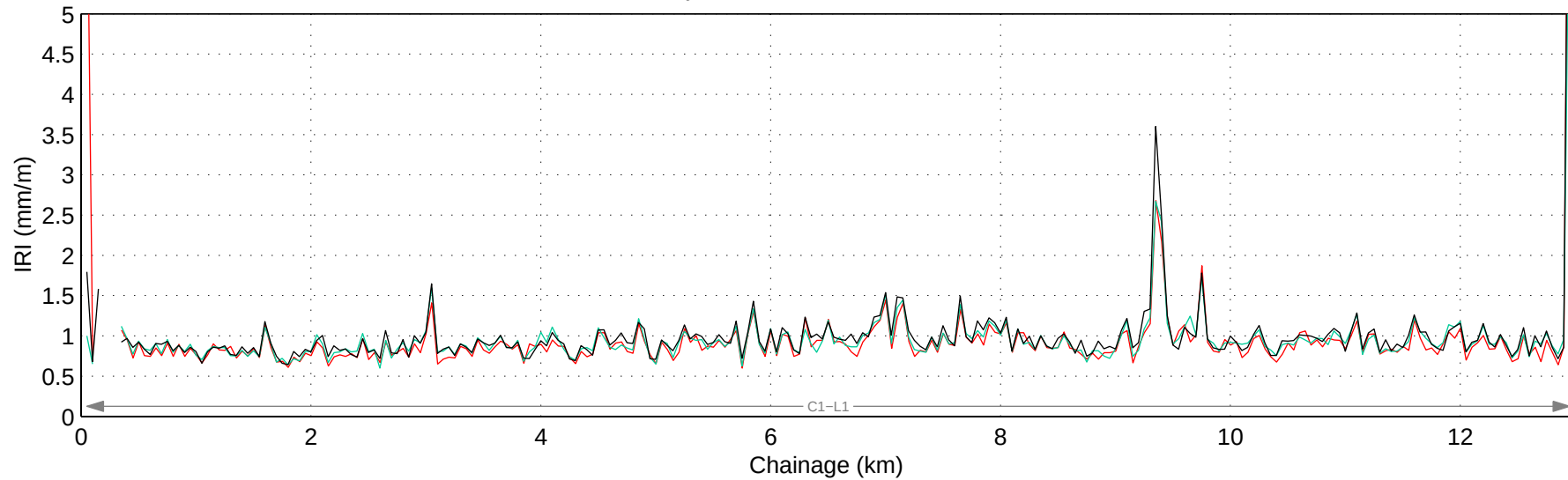
Hwy 771:04 Mean IRI – Left Lane
