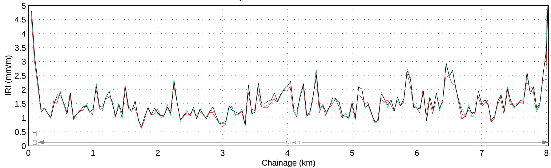
Hwy 775:02 Mean IRI – Left Lane
