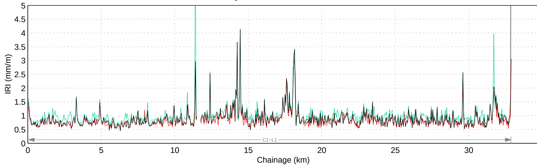
Hwy 722:02 Mean IRI – Left Lane
