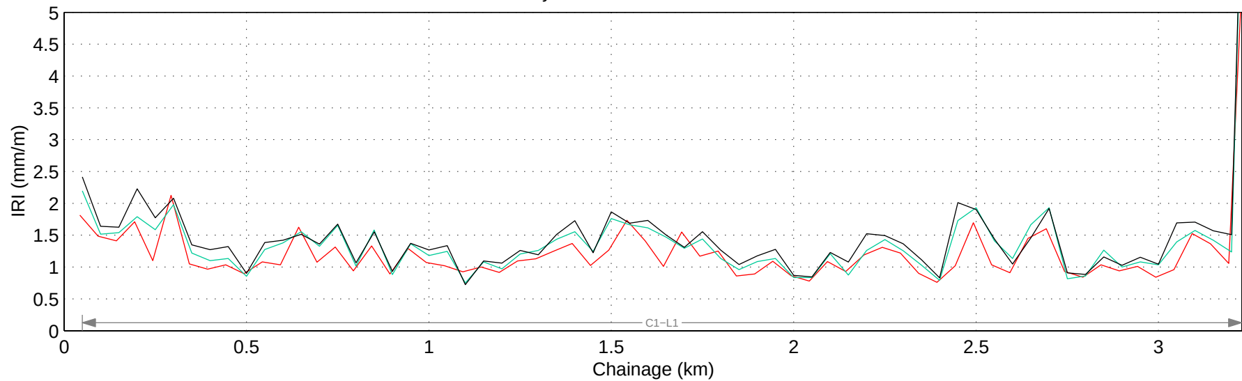
Hwy 782:02 Mean IRI – Left Lane
