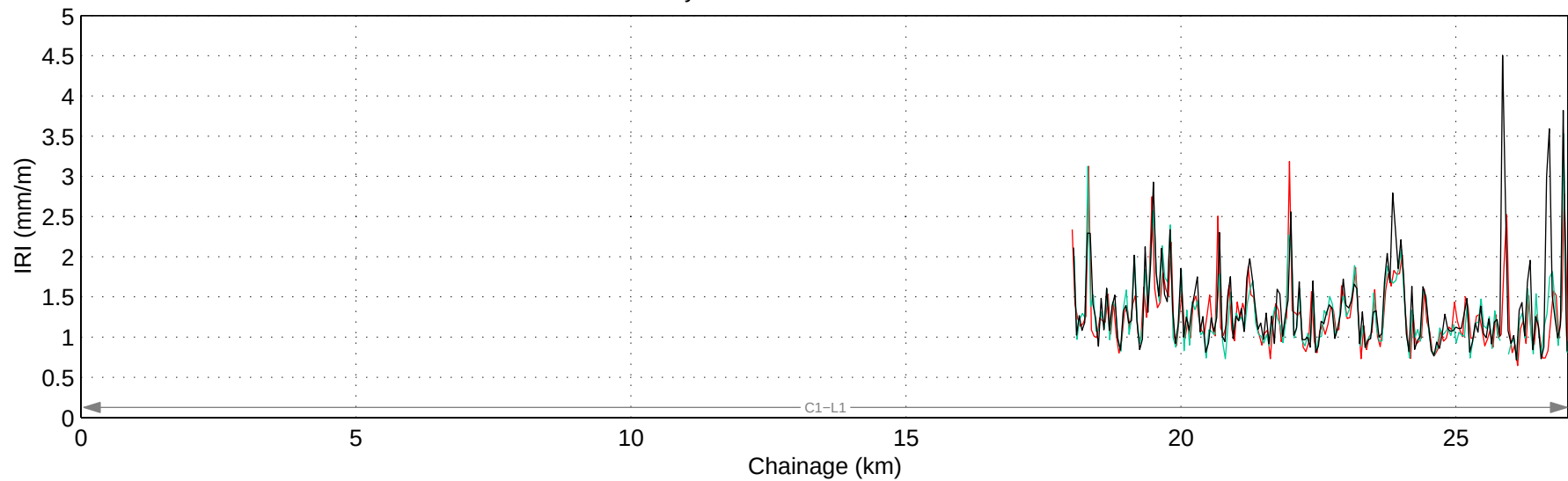
Hwy 752:02 Mean IRI – Left Lane
