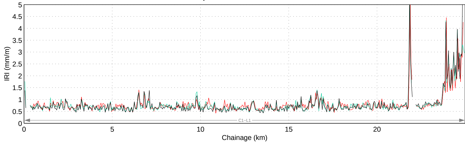
Hwy 781:02 Mean IRI – Left Lane
