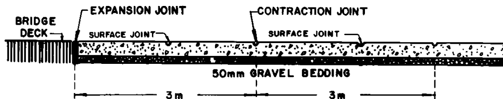
LONGITUDINAL SECTION B-B
