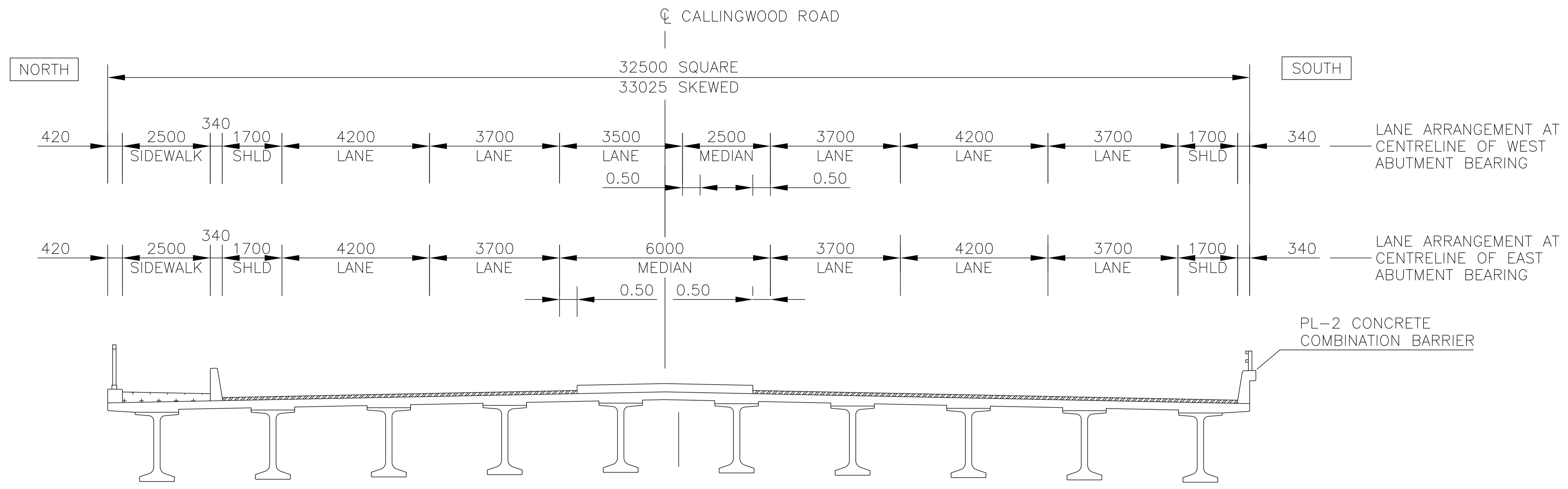
CALLINGWOOD BRIDGE CROSS SECTION (N.T.S.)
