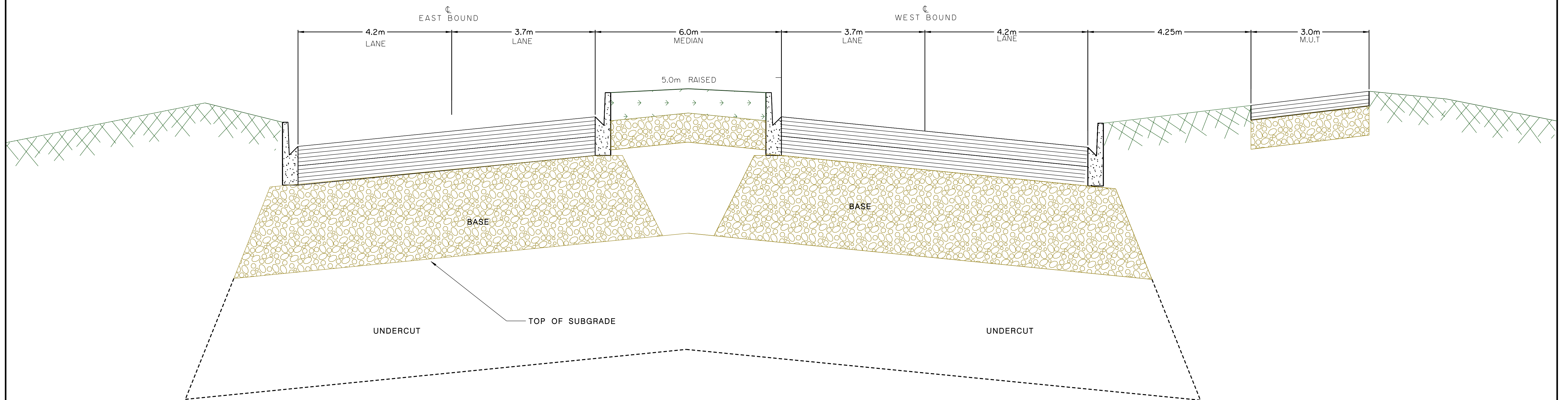
LESSARD ROAD CROSS-SECTION (N.T.S)
