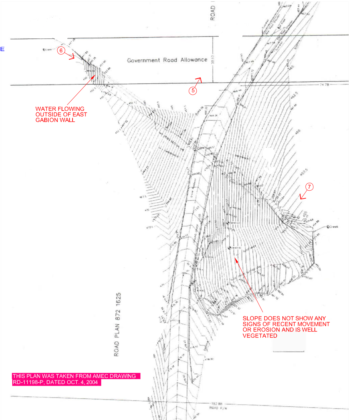
PH11-1 SITE PLAN (STA. 42+600) N.T.S.
