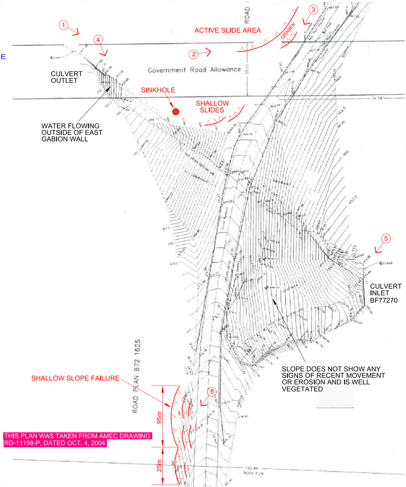
PH11-1 SITE PLAN (STA. 42+600 - BF77270) N.T.S.
