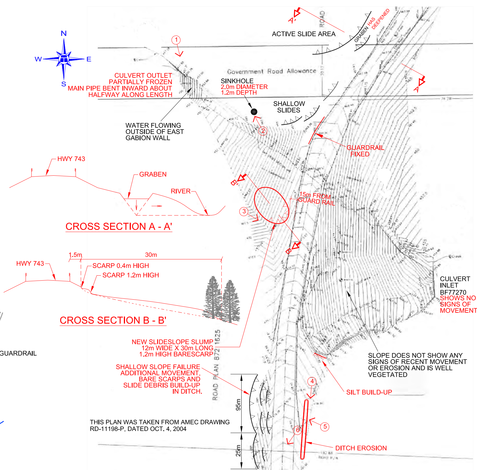
PH11-1 SITE PLAN (STA. 42+600 - BF77270) N.T.S.
