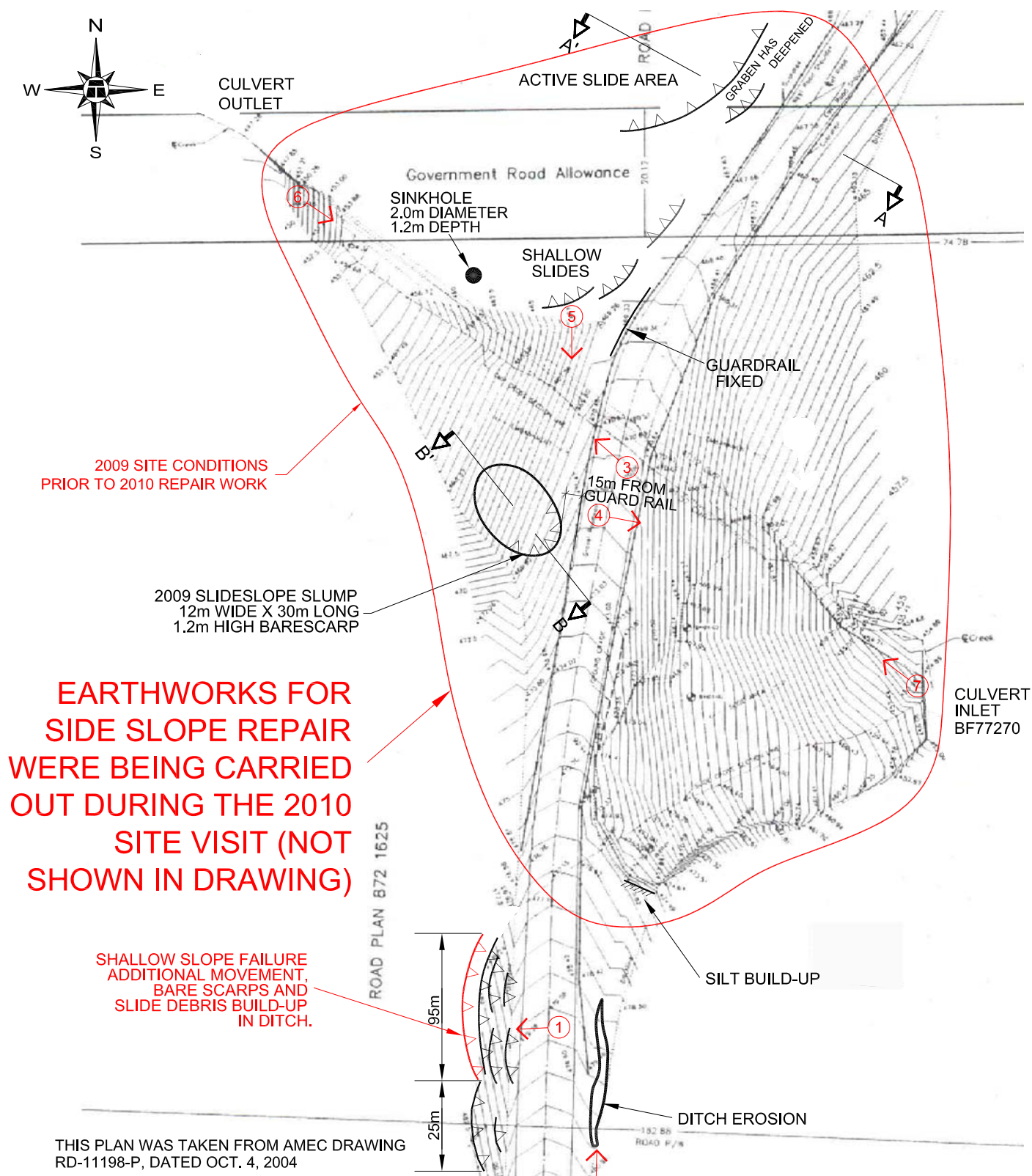
PH11-1 SITE PLAN (STA. 42+600 - BF77270)
