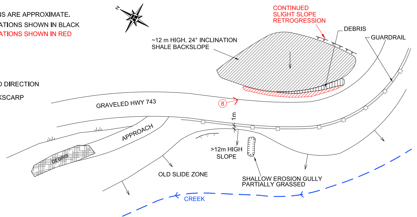
PH11-2 SITE PLAN (STA. 43+200)
