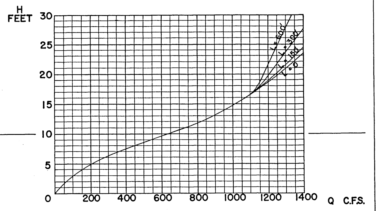
(d) SLOPE 3%
