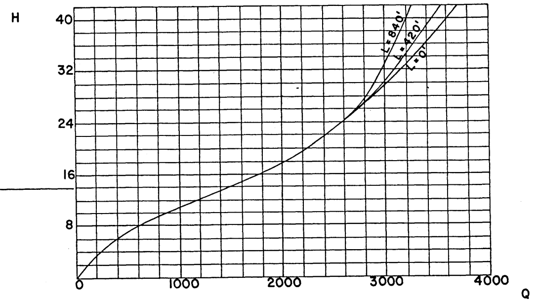
(d) SLOPE 3%
