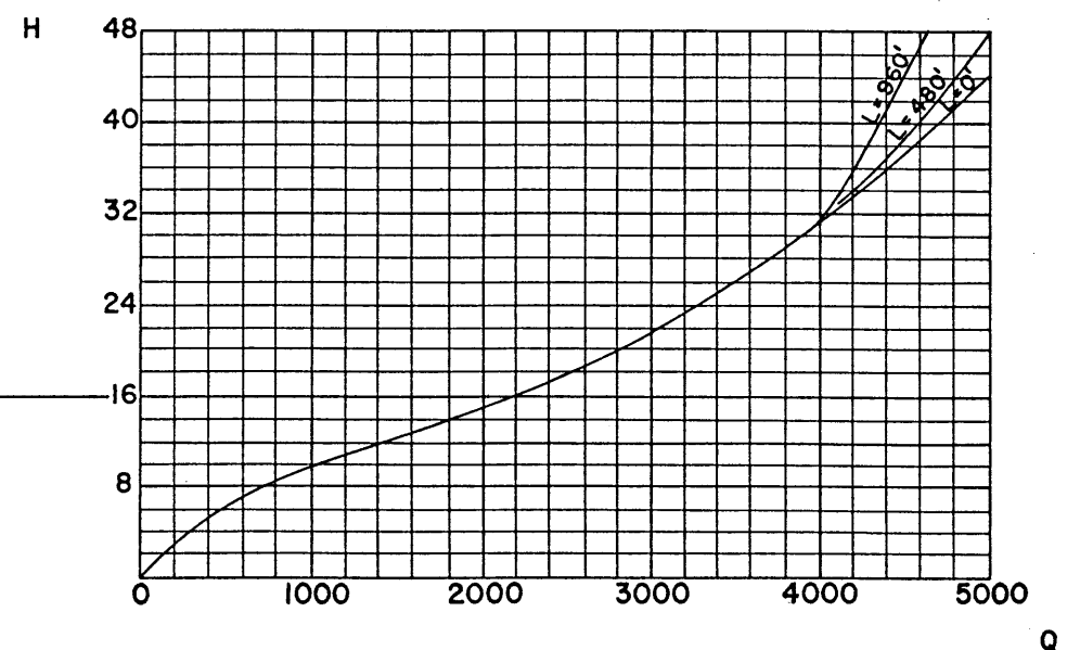
(d) SLOPE 3%
