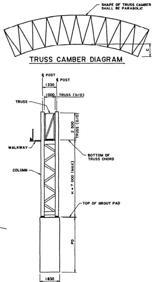
END ELEVATION 1:75
