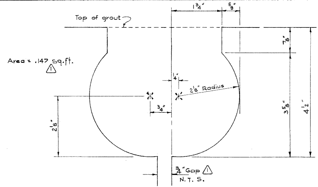
TYPE 'FC' GIRDER Scale: 3/4" = 1"
