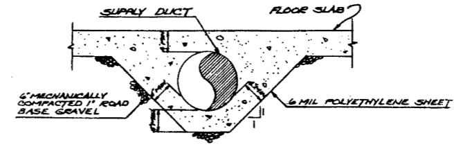
SECTION D N.T.S.
