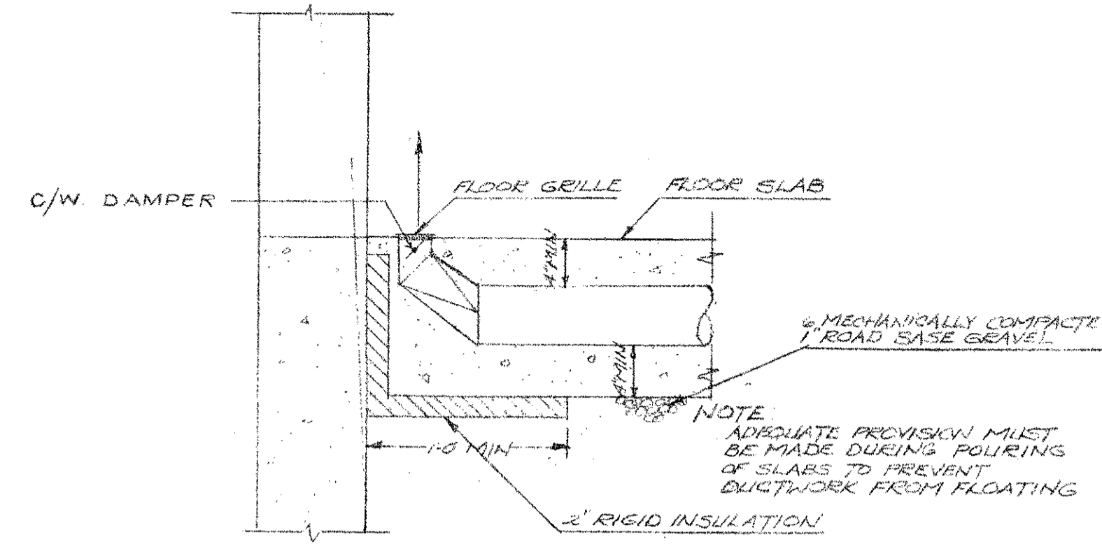
B SECTION SCALE N.T.S.
