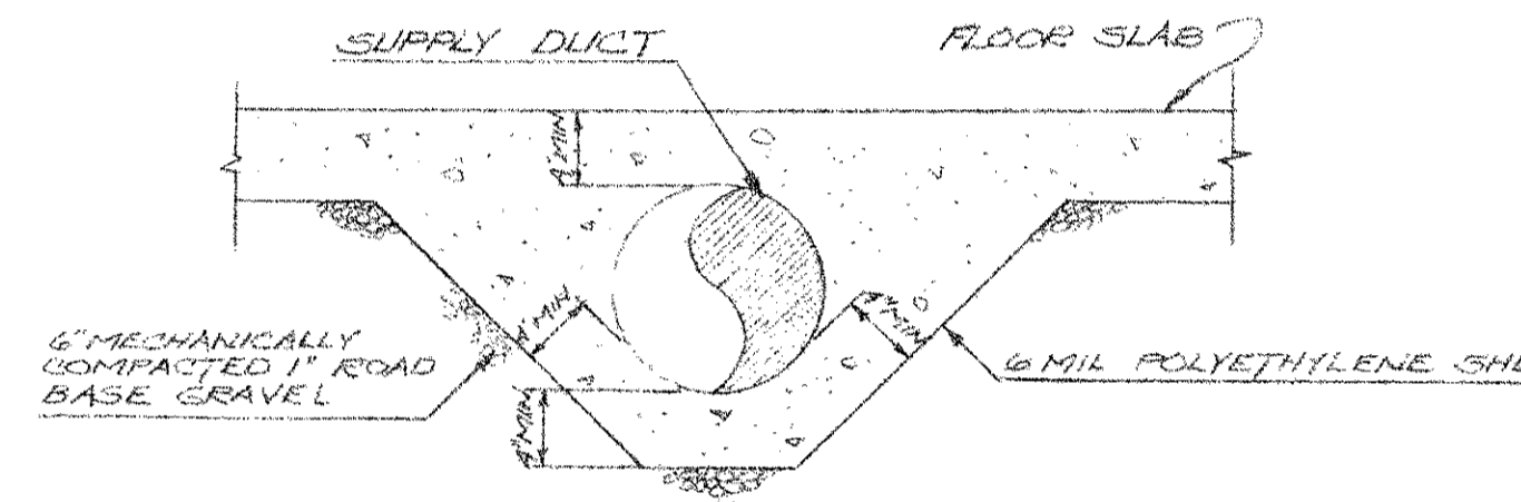
C SECTION SCALE N.T.S.
