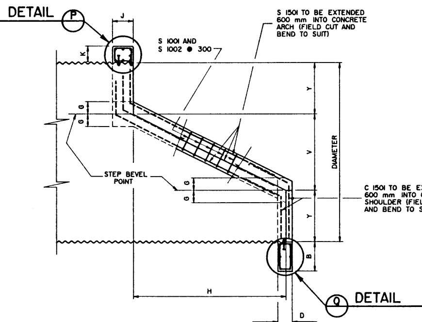
LONGITUDINAL SECTION
